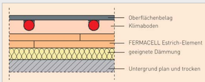
Beispiel 2: Klimaboden auf fermacell Estrich-Element
