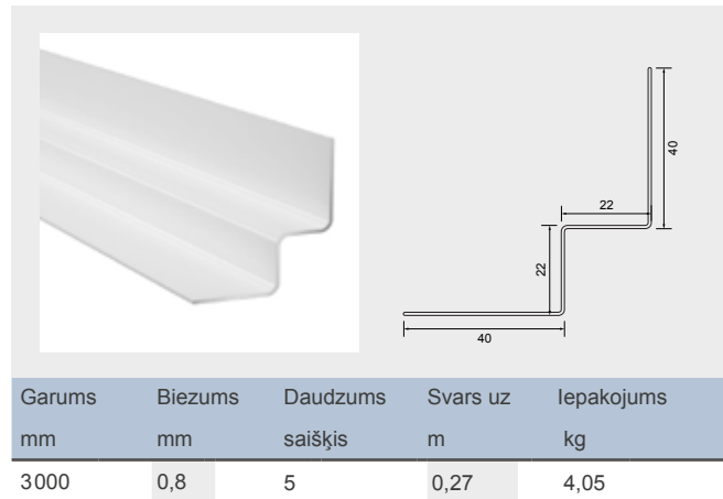
Iekšējā stūra profils
