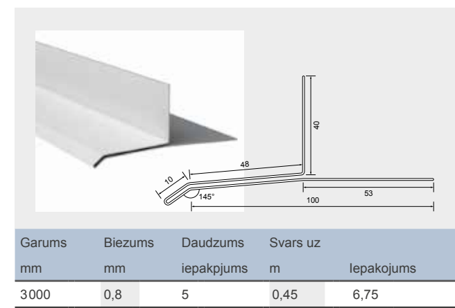
Horizontāla klājuma profils
