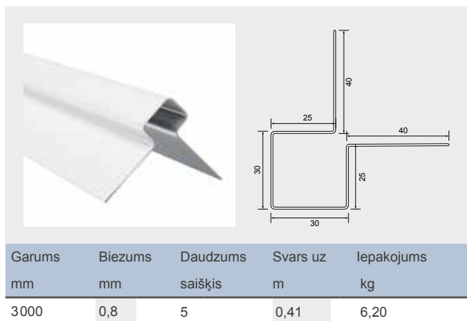
Ārējā stūra profils
